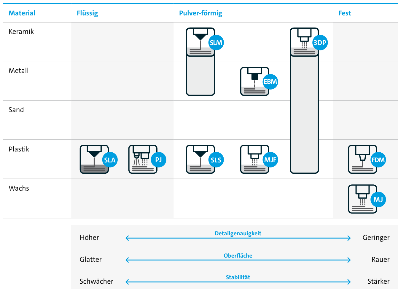
Abbildung 1: Verschiedene 3D-Druck Technologien und ihre Eigenschaften im Überblick 1
